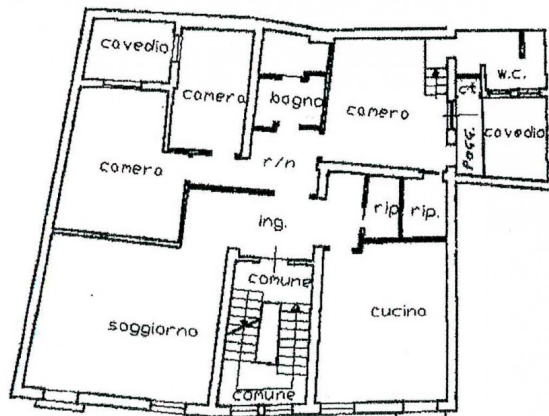
PIANO SECONDO H=290
